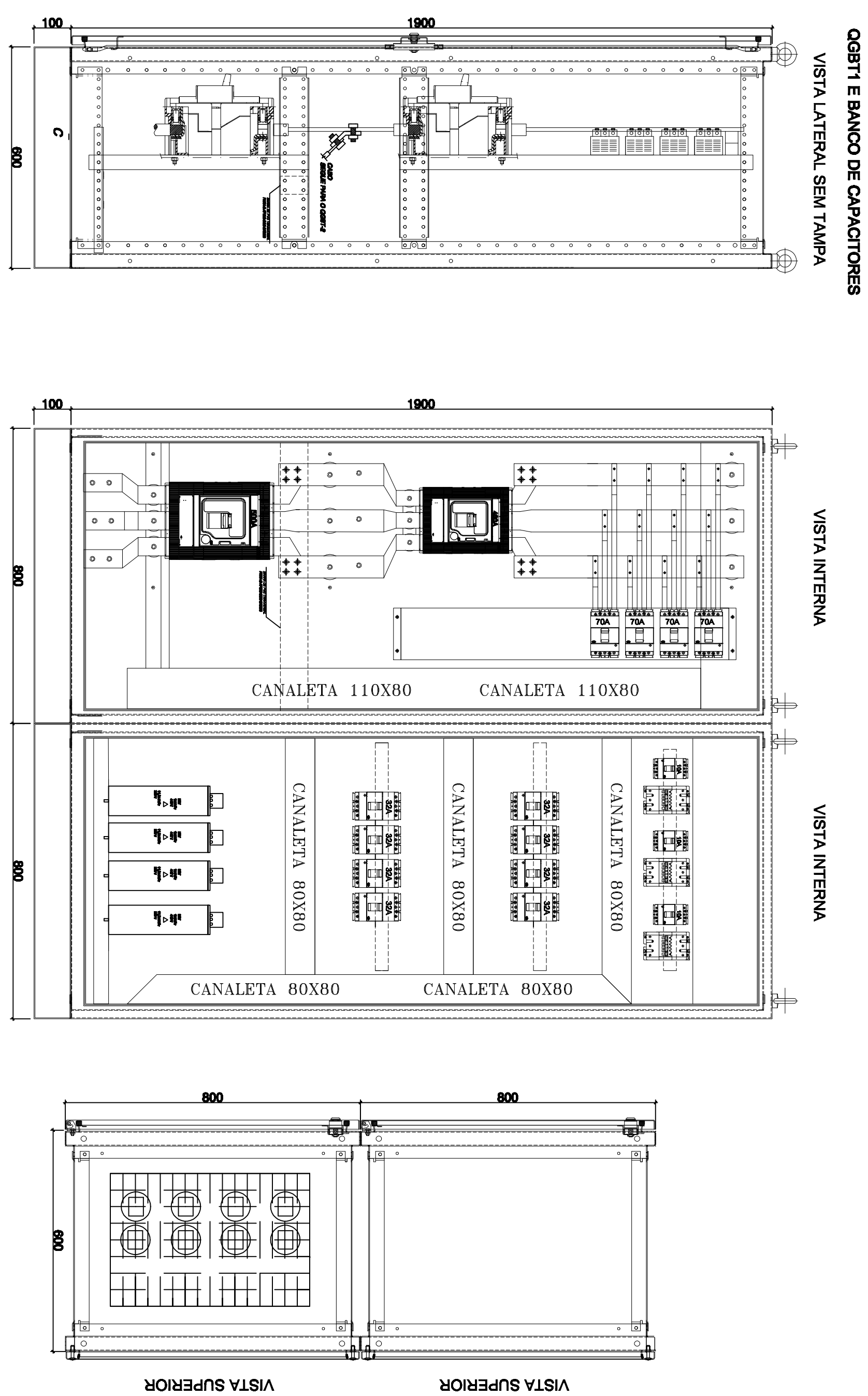
DETALHE DO CABOTE DO BANCO DE CAPACITORES (SUBESTAÇÃO)
