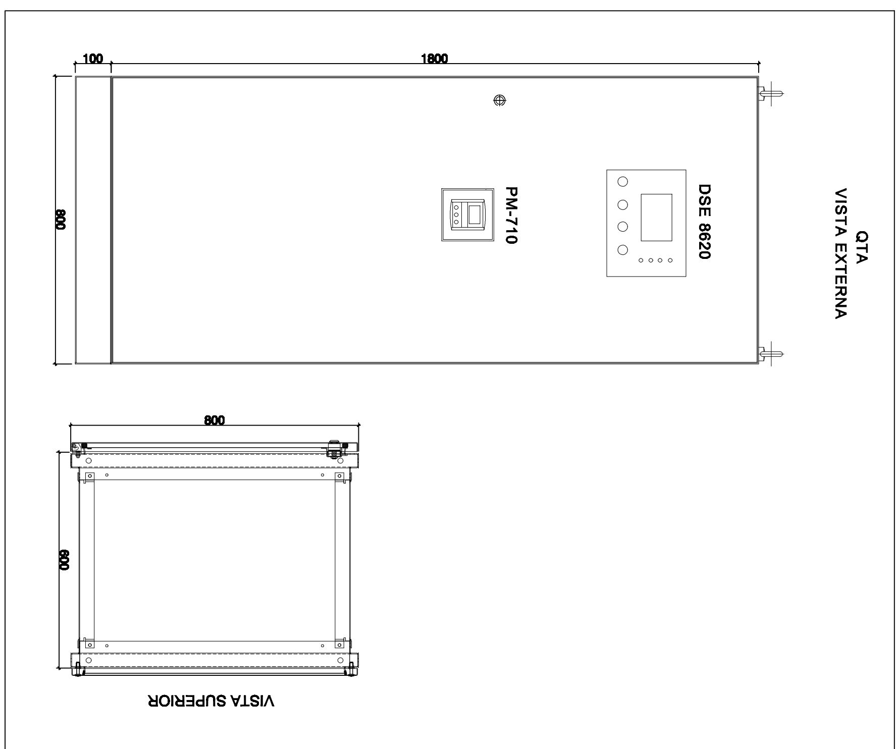
DETALHE DO ORA (QUADRO DE TRANSFERÊNCIA AUTOMÁTICA) Dimensões em mm
